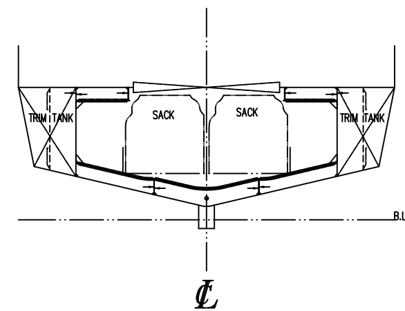
CROSS SECTION FR.7
