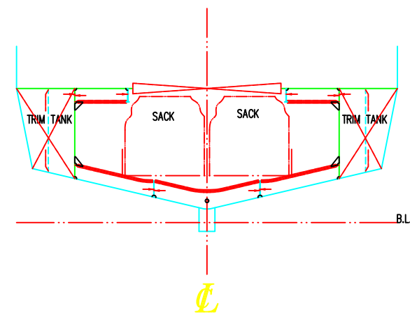
CROSS SECTION FR.7
